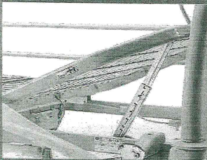
Gambale con movimento a cremagliera Motion of calf section by rack
